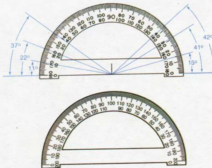
Σχήμα 3.14 Αναγωγείς: α) σε μοίρες (μοιρογνωμόνιο), β) σε βαθμούς (βαθμογνωμόνιο)
