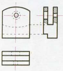
Σχήμα 4.1 Διακεκομμένες γραμμές
