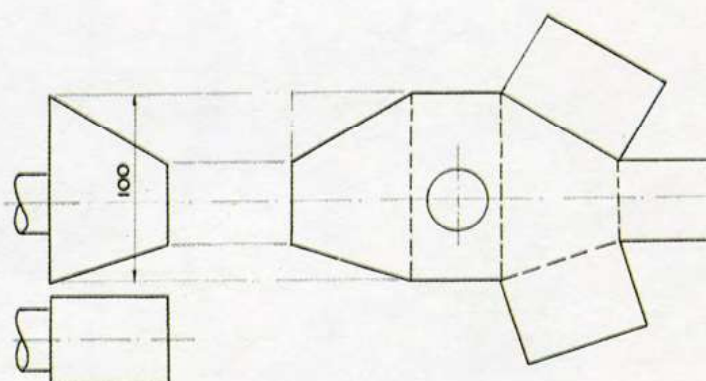
Σχήμα 5.24 ΠΡΙΣΜΑ
