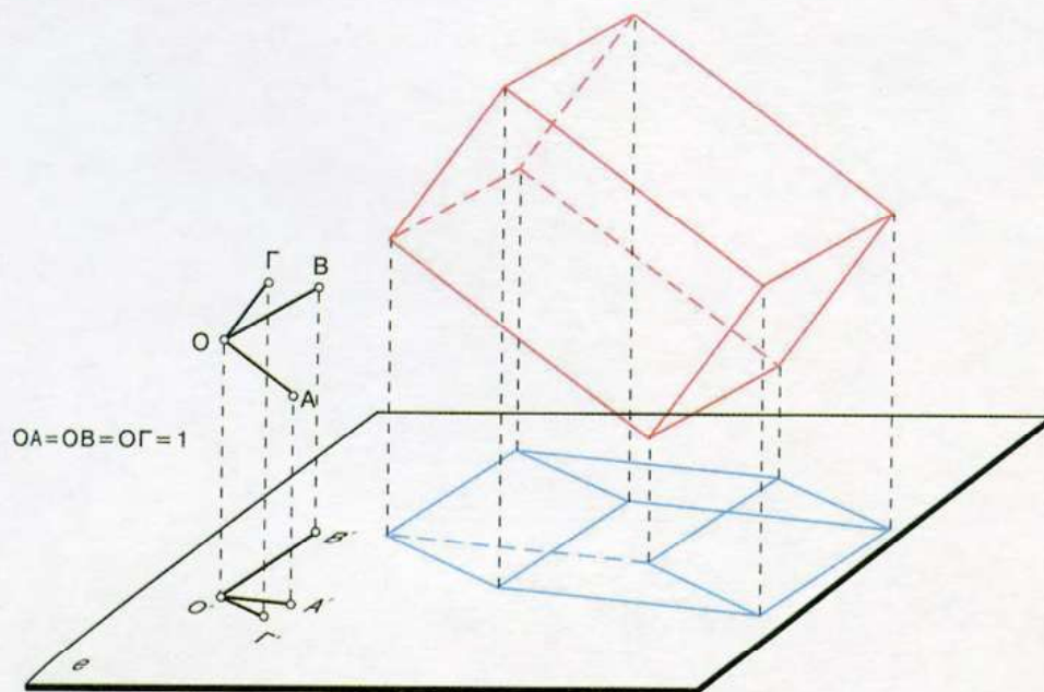
Σχήμα 6.4 Αξονομετρική προβολή παράλληλεπιπέδου
