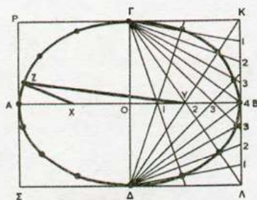
Σχήμα 5.19 Σχεδίαση της έλλειψης
