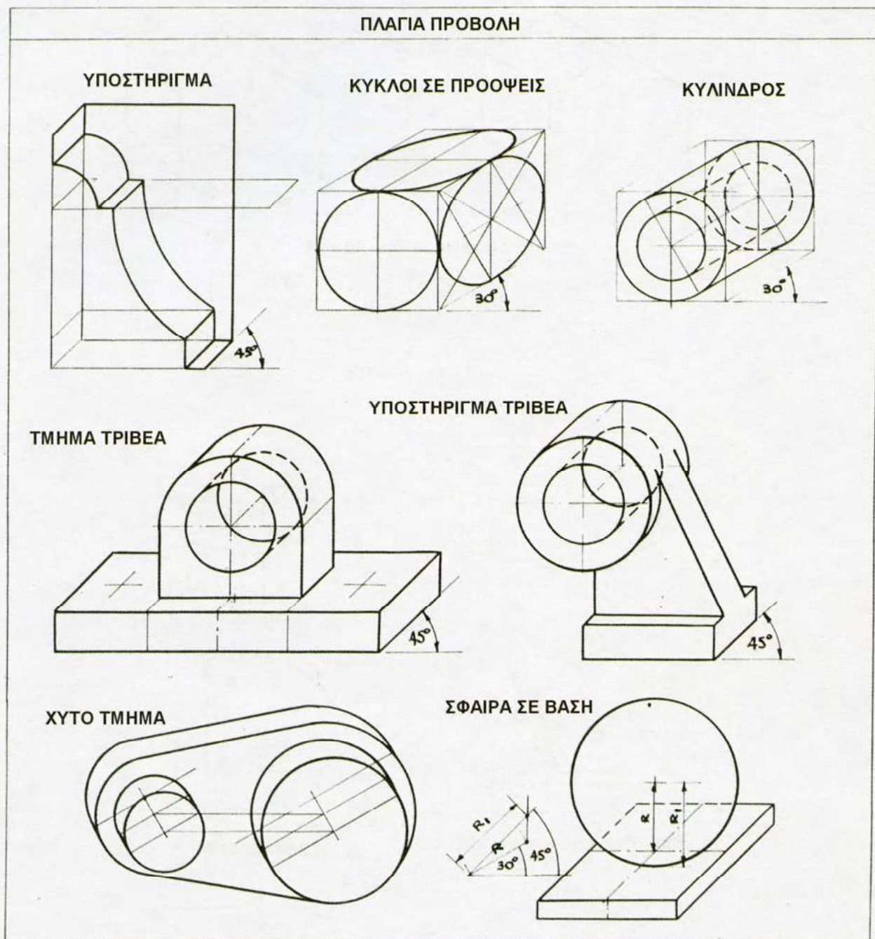
Σχήμα 7.26
