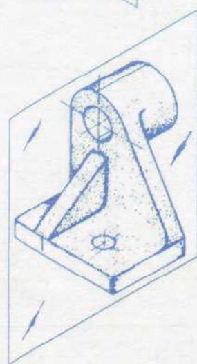
Σχήμα 8.24 Μπρακέτο - Κουζινέτο
