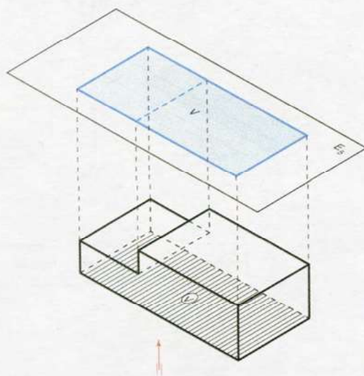
Σχήμα 7.9 Ανοψη
