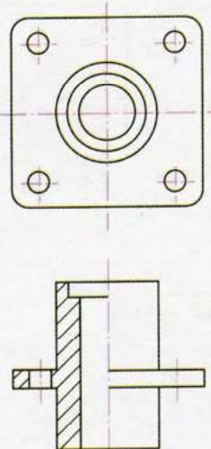
Σχήμα 8.20 Σύνθετη τομή
