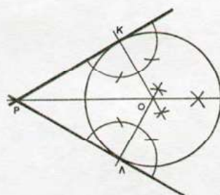
Σχήμα 5.17 Κύκλος στις πλευρές μιας γωνίας
