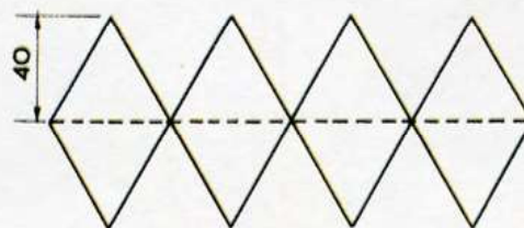
Σχήμα 5.22 ΑΝΑΠΤΥΓΜΑ ΟΚΤΑΕΔΡΟΥ
