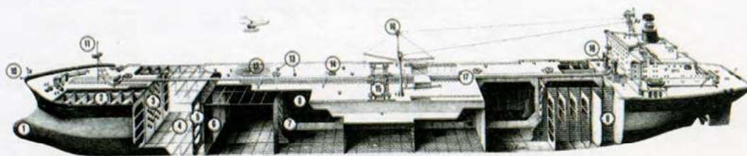
Σχήμα 9.13 Λεπτομέρειες ενός δεξαμενοπλοίου
