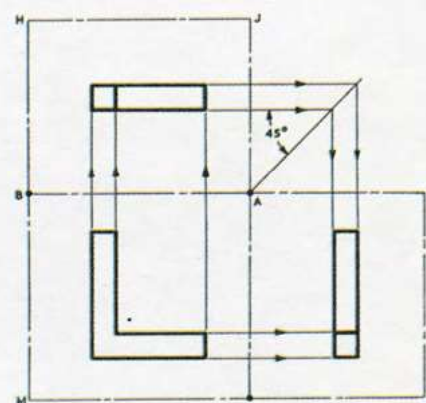
Σχήμα 7.33 Η τρίτη γωνία ορθογραφικής προβολής
