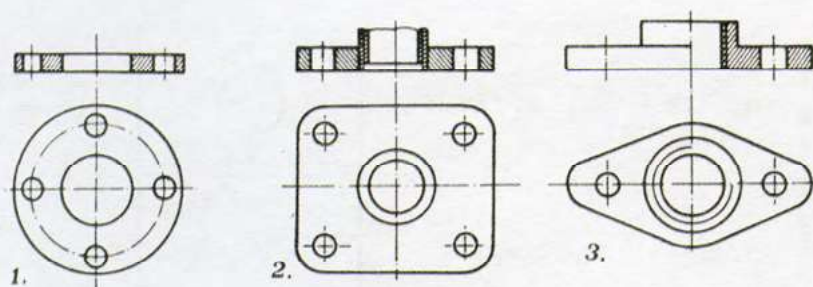
Σχήμα 9.1 Τύποι φλαντζών
