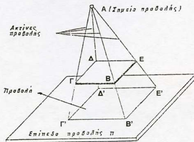
Σχήμα 6.1 Κεντρική προβολή
