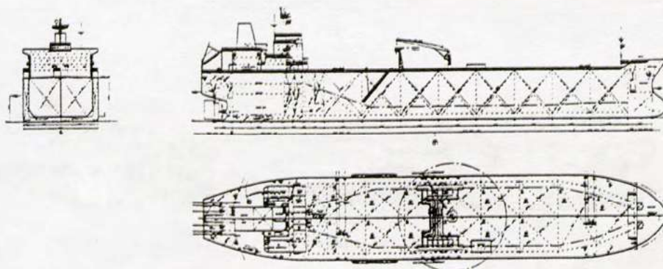
Σχήμα 9.8 Chemical carrier
