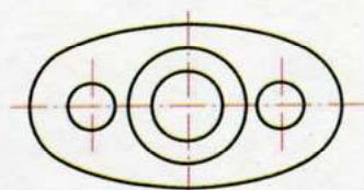
Κάτοψη
