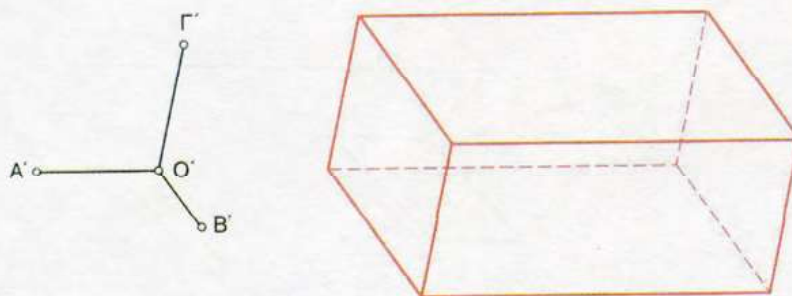
Σχήμα 6.5 Αξονομετρική προβολή των τριών μονάδων και του ορθογώνιου παράλληλεπιπέδου
