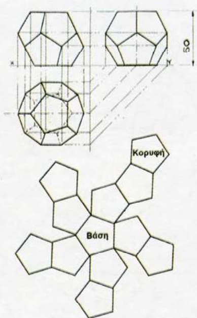
Σχήμα 5.23 ΔΩΔΕΚΑΕΔΡΟ
