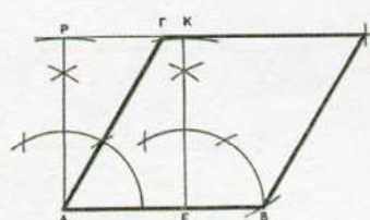
Σχήμα 5.12 Σχεδίαση παραλληλογράμμου
