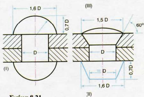
Σχήμα 8.21 Καρφωτά ελάσματα
