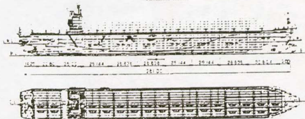
Σχήμα 9.9 Containership
