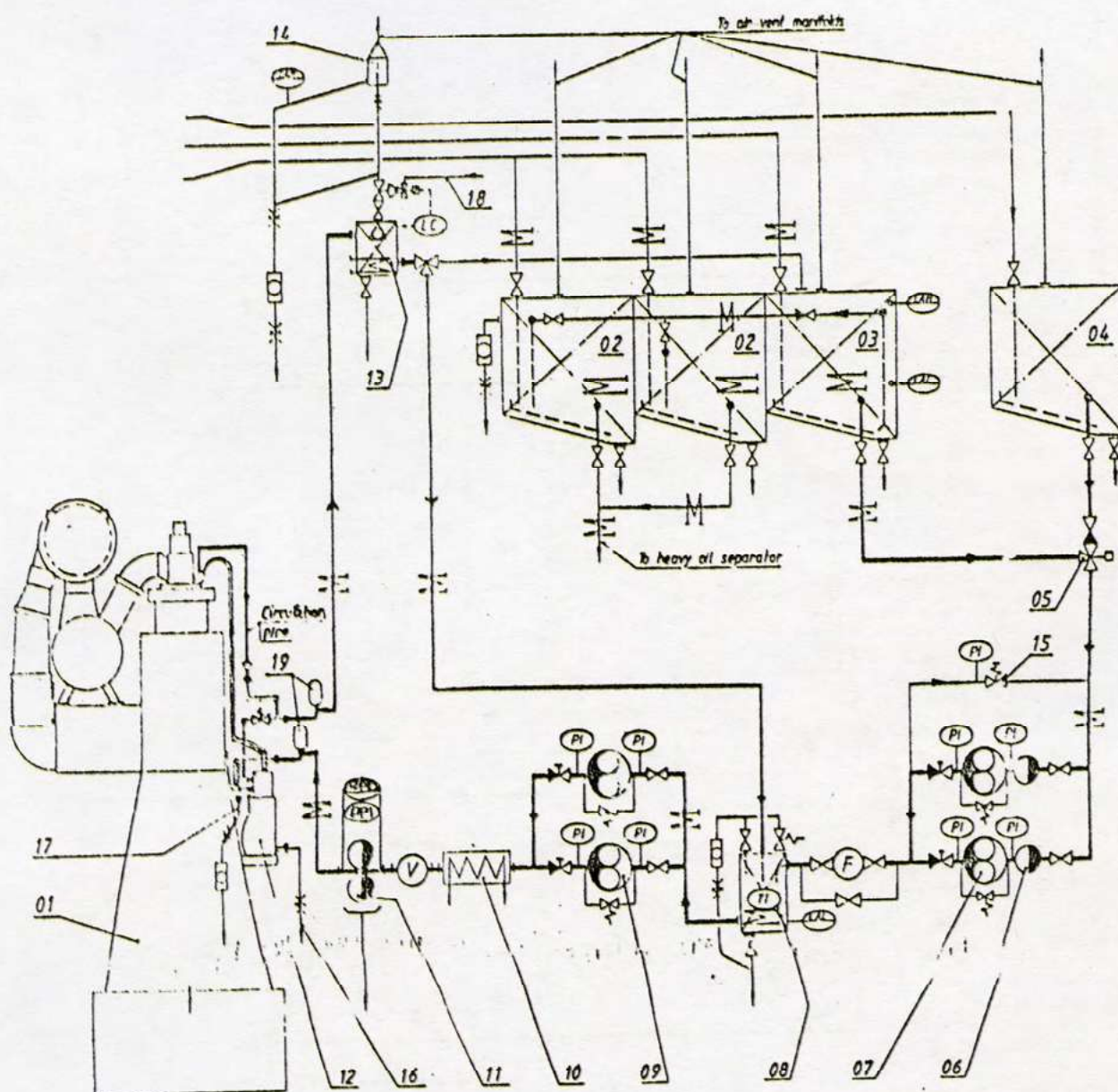
Σχήμα 9.17 Δίκτυο καυσίμων
