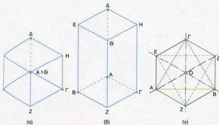
Σχήμα 6.6 Αξονομετρική προβολή: α) κύβου, β) πρίσματος με τετράγωνη βάση και ύψος διπλάσιο από την ακμή της βάσης, γ) κανονικού οκταέδρου.
