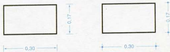
Σχήμα 4.3 Γραμμές διαστάσεων
