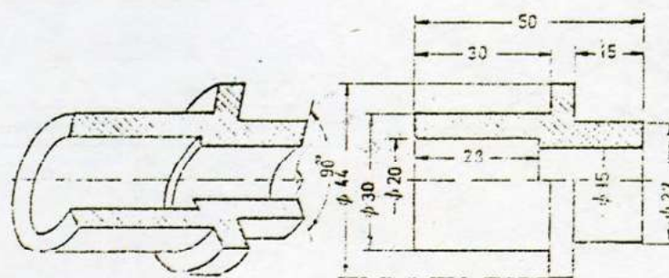
Σχήμα 8.4 Ημιτομή
