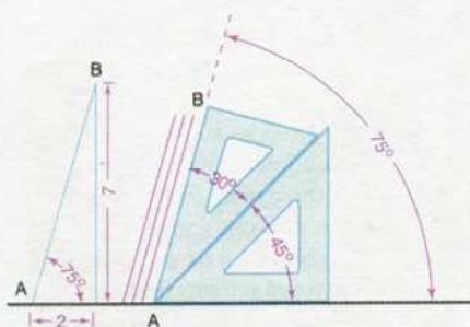
Σχήμα 4.5 Κατασκευή οδηγητικών γραμμών για λοξά γράμματα
