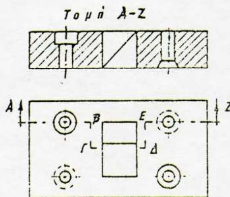
Σχήμα 8.20 Σύνθετη τομή
