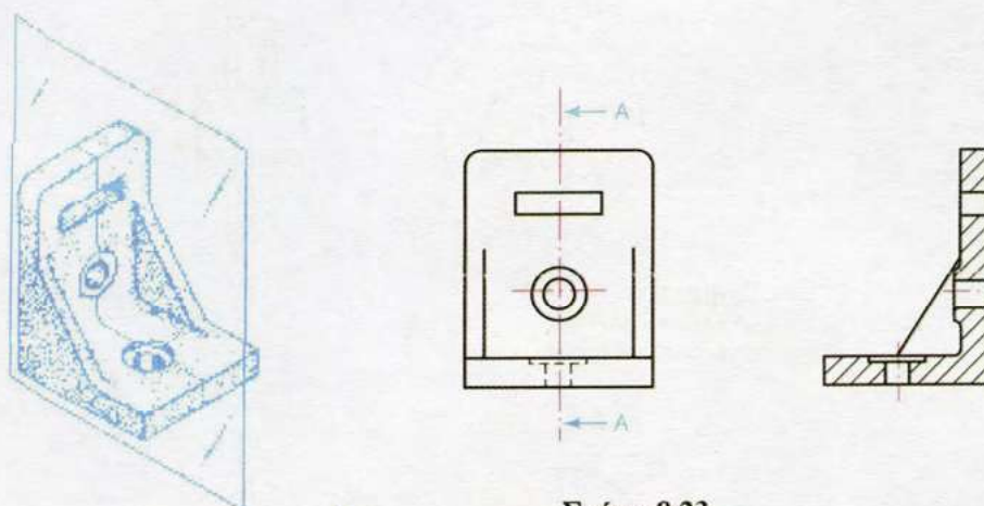
Σχήμα 8.23 Γωνία στήριξης
