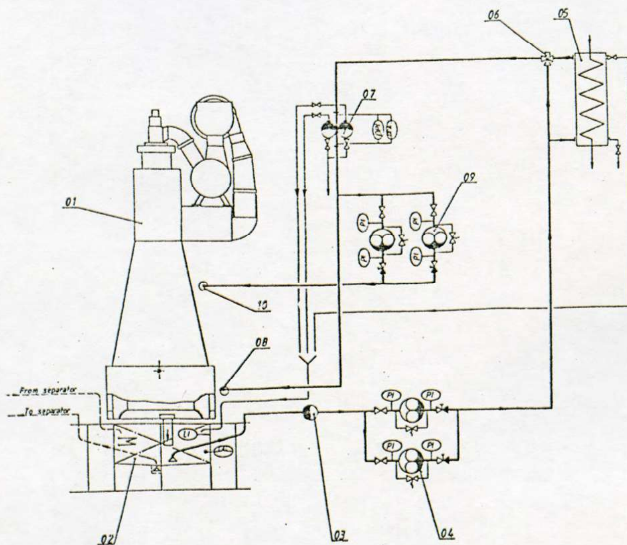
Σχήμα 9.19 Δίκτυο λίπανσης
