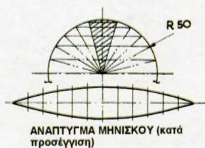
Σχήμα 5.26 ΣΦΑΙΡΑ
