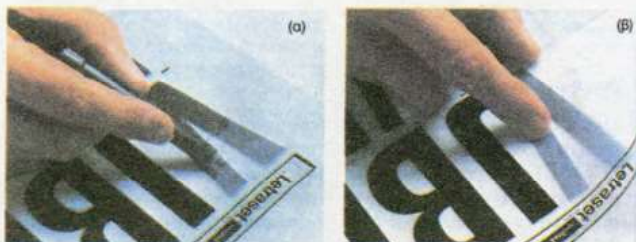
Σχήμα 4.11 Επικόλληση γραμμάτων: α) με σπάτουλα, β) με το δάκτυλο
