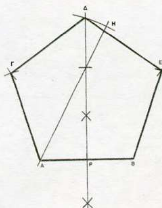
Σχήμα 5.15 Κανονικό πεντάγωνο
