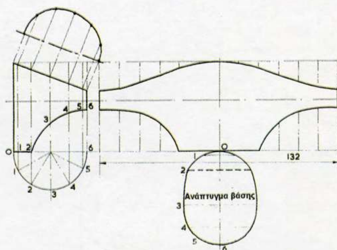
Σχήμα 5.25 ΚΥΛΙΝΔΡΟΣ
