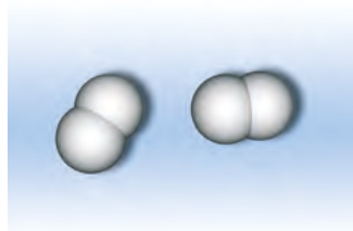
Τα μόρια του υδρογόνου μετά τη διάσπαση
