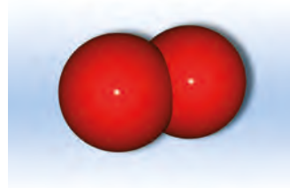
Το μόριο του οξυγόνου μετά τη διάσπαση
