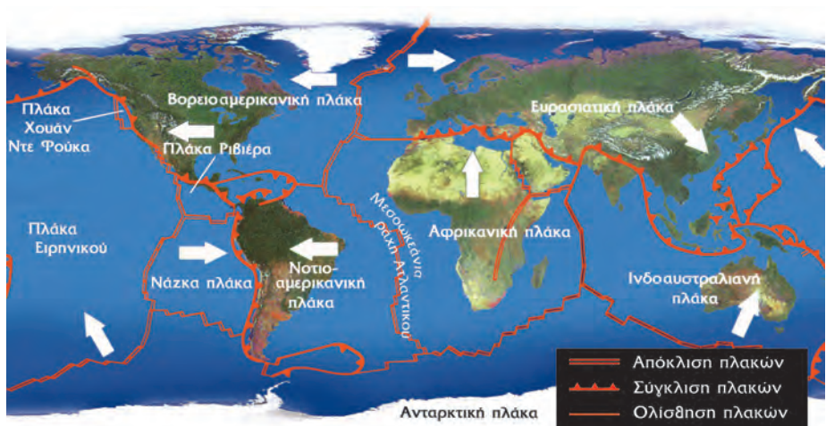
6.3 Κινήσεις λιθοσφαιρικών πλακών
