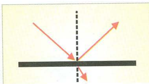
Σχήμα 25: Διάθλαση
