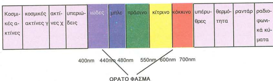
Σχήμα 23: Φάσμα φωτός
