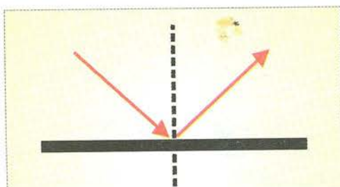
Σχήμα 24: Ανάκλαση
