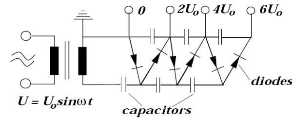
Κύκλωμα Greinacker
