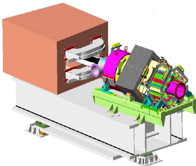
Διάταξη υμκυψέλης του δακτυλίου του SNS
