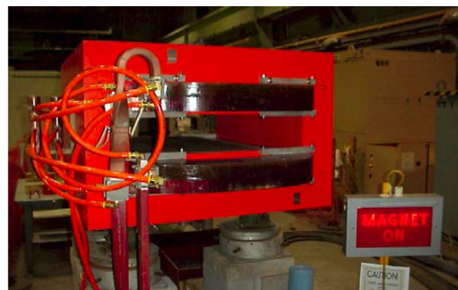
Δίπολο του δακτυλίου του SNS
