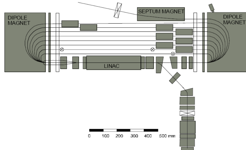
Μίκροτρον του MAMI σε σχήμα σταδίου
