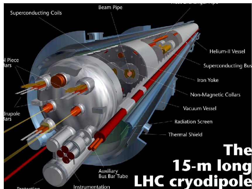
Υπεραγώγιμο δίπολο του LHC
