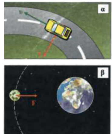
Εικ. 1.12 Δυνάμεις που δρουν ως κεντρομόλες: α) η τριβή, β) η βαρυτική έλξη F .
