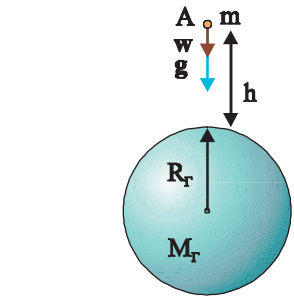
Σχ. 5.52 Το σημείο A βρίσκεται σε ύψος h , πάνω από την επιφάνεια της Γης.
