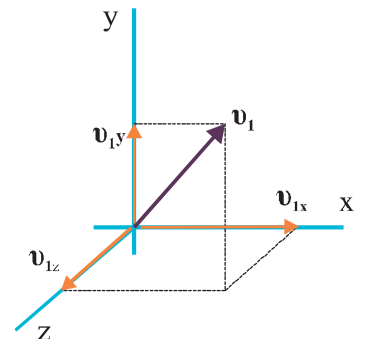
Σχ. 3.8 Η ταχύτητα αναλύεται σε τρεις συνιστώσες σε τρισσορθόγωνιο σύστημα συντεταγμένων.
