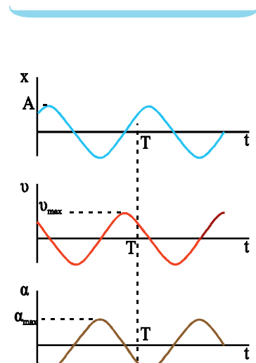
Τα διαγράμματα της απομάκρυνσης, της ταχύτητας και της επιτάχυνσης σε μια ταλάντωση με αρχική φάση.
