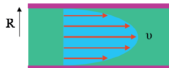
Διάγραμμα ταχυτήτων για ένα ρευστό σε κυλινδρικό σωλήνα ακτίνας R .
