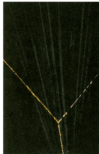
Δύο σωματίδια \alpha συγκρούονται. Το ένα, πριν την κρούση, ήταν πρακτικά ακίνητο.
