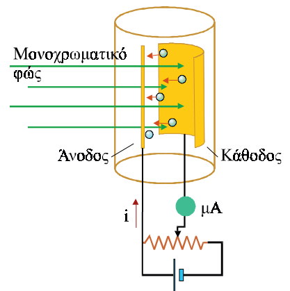
Σχηματική παράσταση ενός κυκλώματος φωτοκύτταρου.
