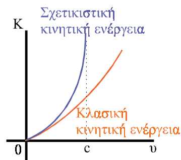
Παρατηρούμε ότι για v \ll c οι δυο καμπύλες πρακτικά συμπίπτουν.
