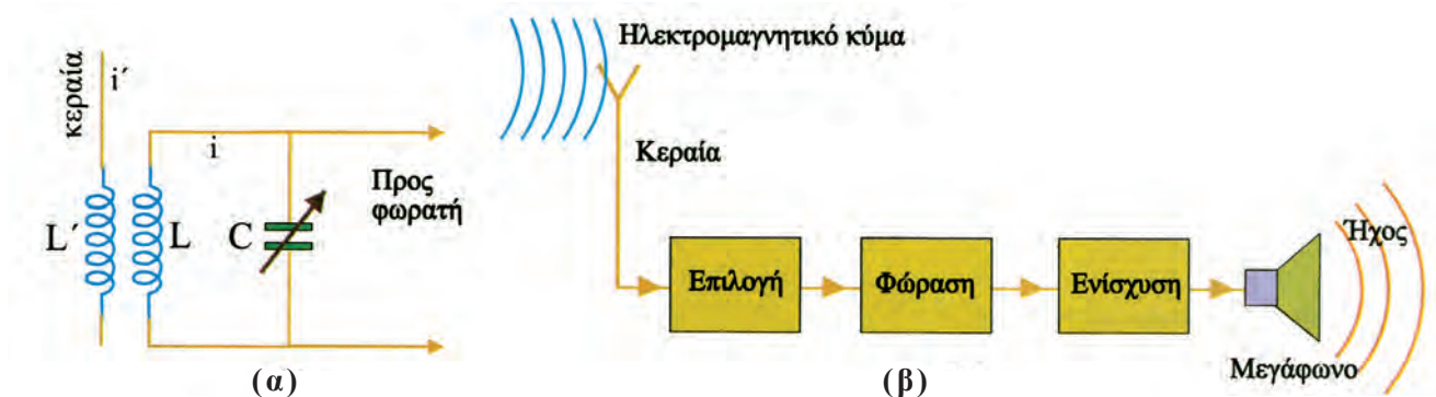
(α) Το κύκλωμα επιλογής (β) Σχηματική παράσταση της διαδικασίας λήψης
