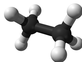
Μοντέλο δομής για την ένωση C_2H_6 .
