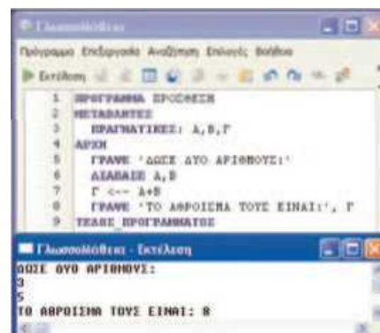
Εικόνα 1.4. Ο κώδικας για την άθροιση δύο αριθμών στο προγραμματιστικό περιβάλλον Γλωσσολόβη.
