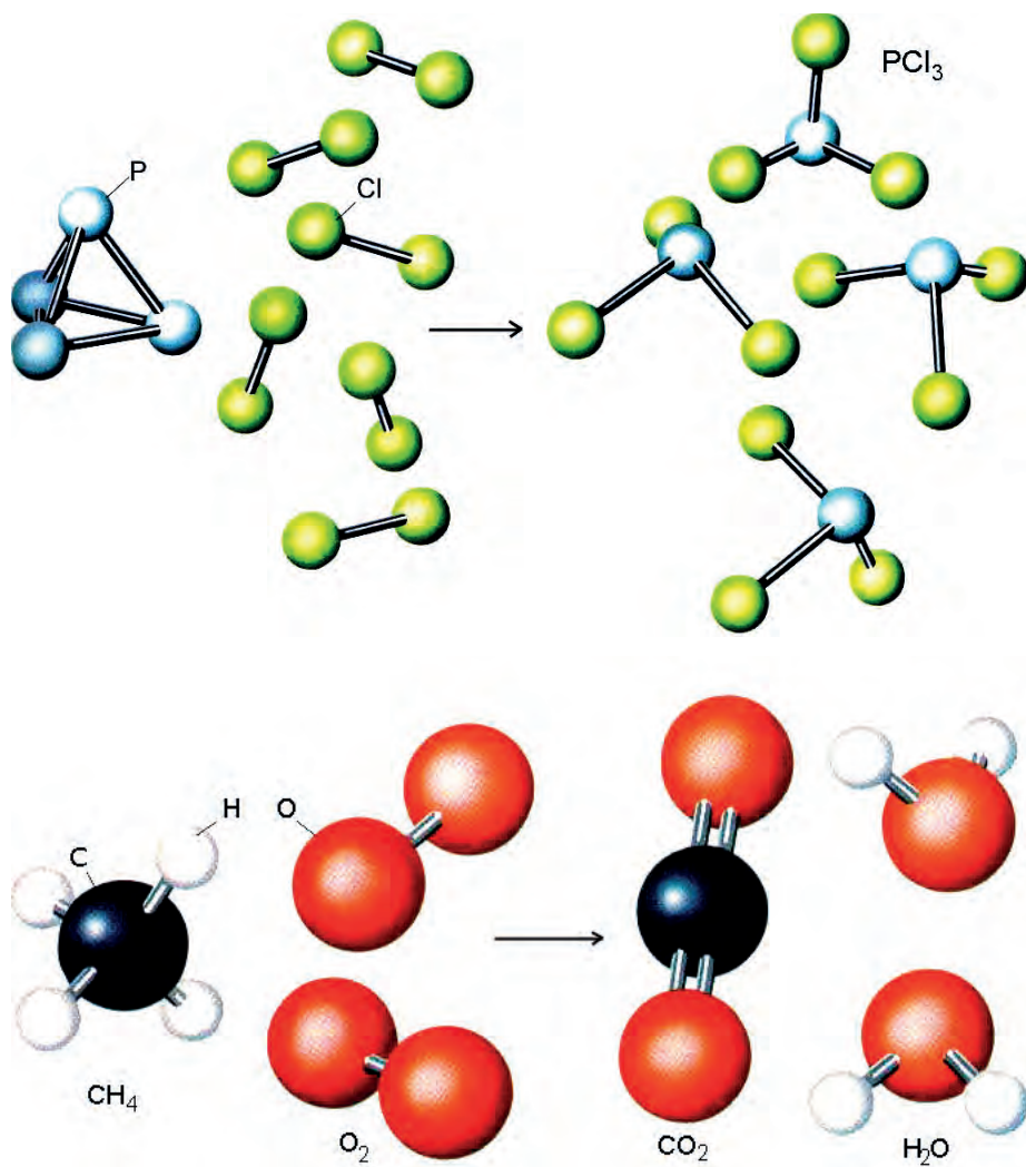
ΣΧΗΜΑ 3.7 Εικονική παρουσίαση των αντιδράσεων σε μορφή μοριακών μοντέλων : α. \text{P}_4(\text{s}) + 6\text{Cl}_2(\text{g}) \rightarrow 4\text{PCl}_3(\text{s}) (πάνω) β. \text{CH}_4(\text{g}) + 2\text{O}_2(\text{g}) \rightarrow \text{CO}_2(\text{g}) + 2\text{H}_2\text{O}(\text{g}) (κάτω).
