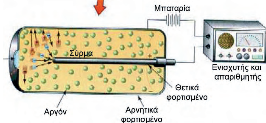
ΣΧΗΜΑ 5.5 Αρχή λειτουργίας του μετρητή Geiger – Muller. Η ραδιενεργός ακτινοβολία εισέρχεται στο θάλαμο και ionτίζει τα άτομα ενός ευγενούς αερίου. Έτσι, παράγεται ηλεκτρικό ρεύμα το οποίο αφού ενισχυθεί καταγράφεται.
