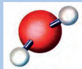
μόριο H 2 O
