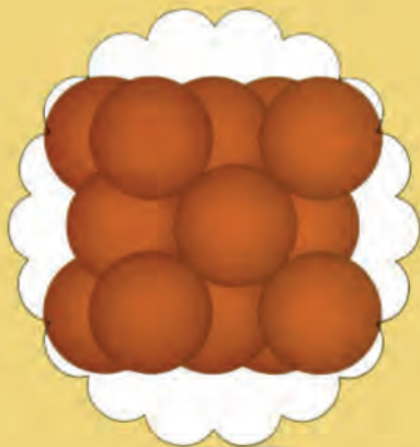
Άτομα
