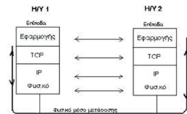
Εικόνα 9.2. Η λειτουργία του πρωτοκόλλου TCP/IP
