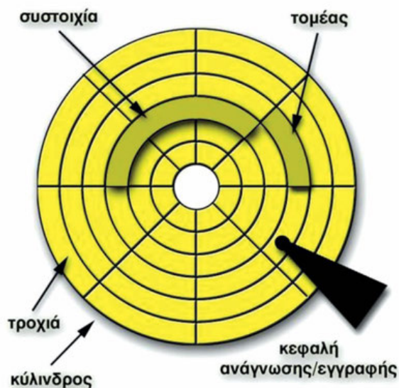
Εικόνα 2.5: Φυσική οργάνωση του μέσου αποθήκευσης. (πηγή: βιβλιογραφία #9)
