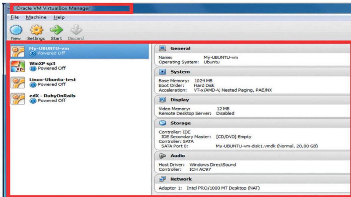
Εικόνα 6.1: Πρόγραμμα Επόπτη με Εικονικές Μηχανές
