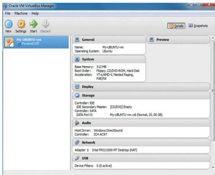
Παράρτημα 2 – Εικόνα 8 – Εικόνα Επόπτη με VM
