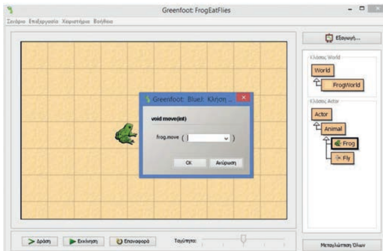
Εικόνα 2.4.2 Κλήση μεθόδου
