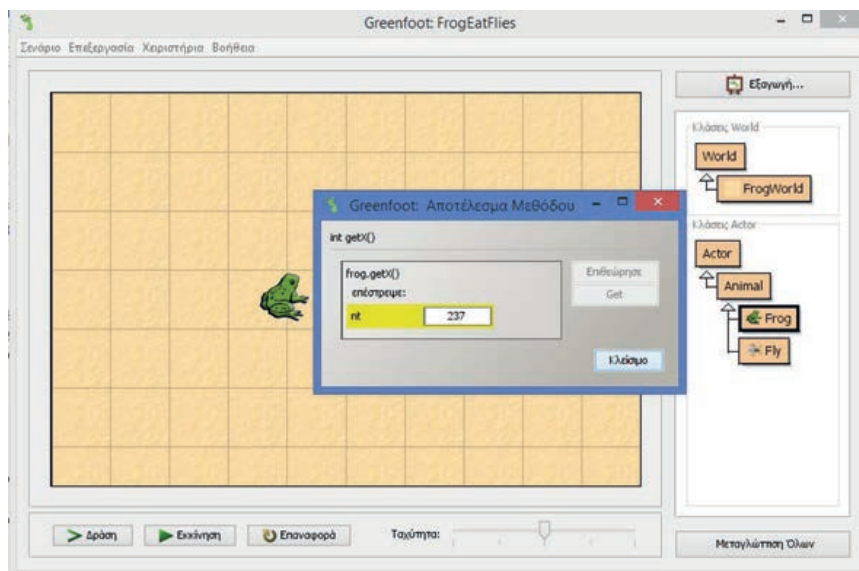
Εικόνα 2.4.3 Αποτέλεσμα μεθόδου
