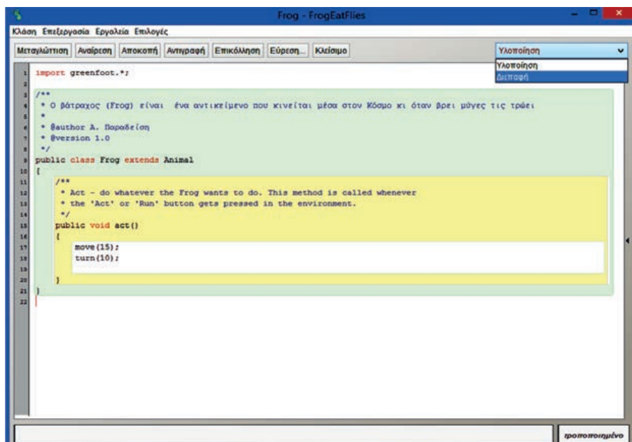
Εικόνα 2.5.5 Εισαγωγή σχολίων
