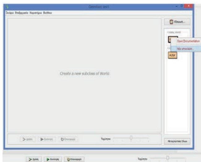
Εικόνα 1.5.3 Δημιουργία υποκλάσης
