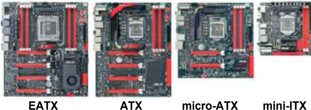
Εικόνα 8: Μητρικές πλακέτες
