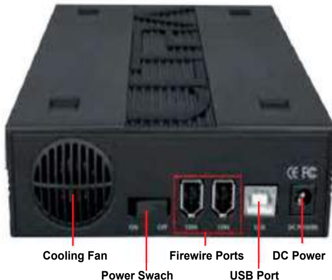
Εικόνα 49: Firewire Ports
