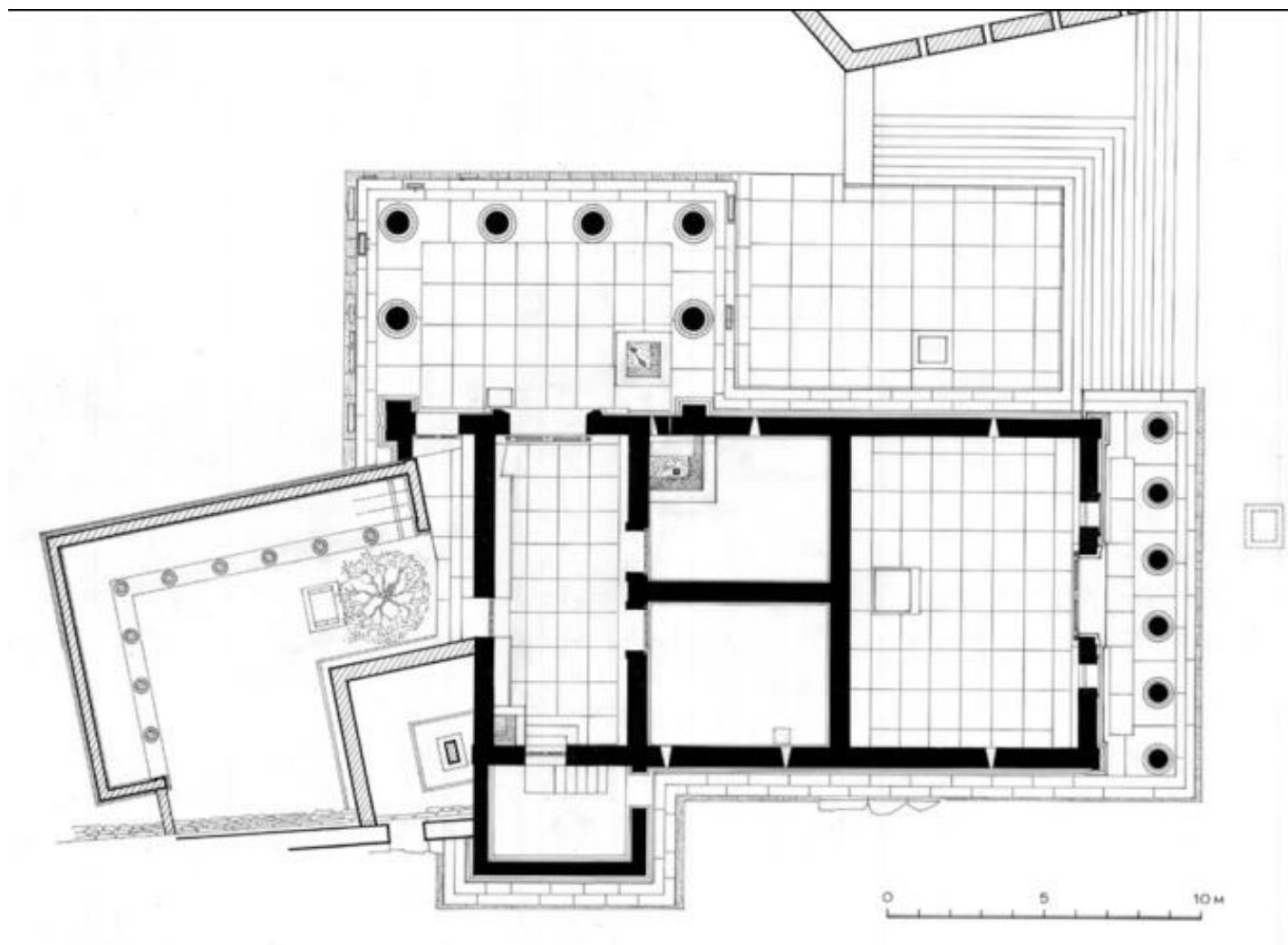
Κάτοψη Ερέχθειο
