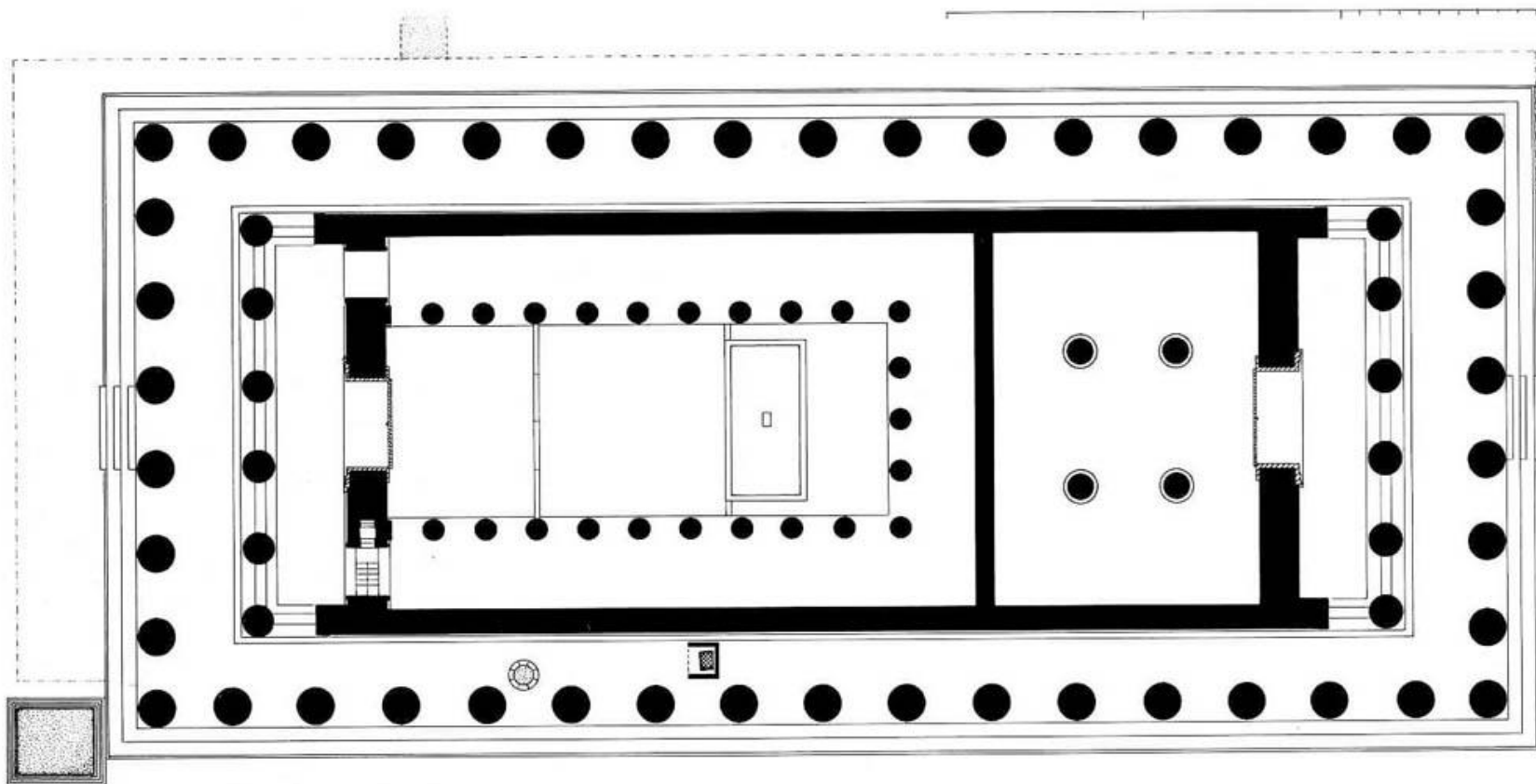
Κάτοψη του Παρθενώνα
