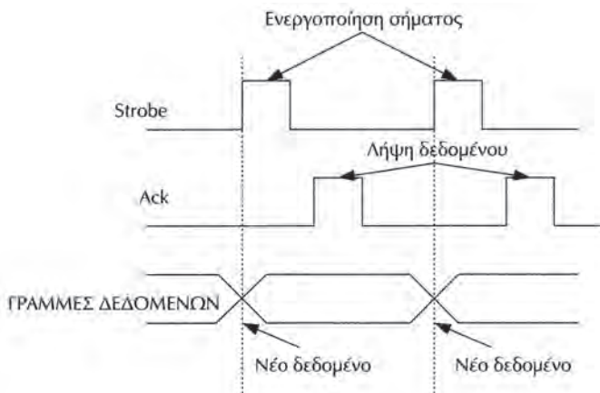
Σχήμα 3.9.2 Απλή χειραψία
