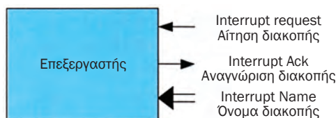
Σχήμα 3.8.2 Σήματα διακοπών
