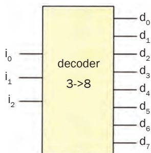
Σχήμα 3.7.5 Σχηματικό αποκωδικοποιητή
