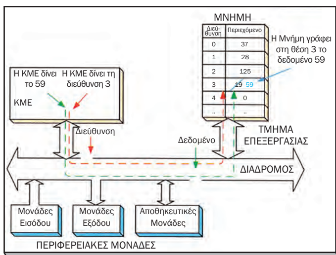
Σχήμα 3.1.10 Εγγραφή στη μνήμη
