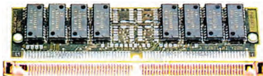
Σχήμα 4.5.5 Μνήμη σε συσκευασία SIMM 72 επαφών και η αντίστοιχη βάση.
