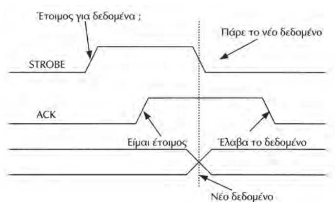
Σχήμα 3.9.4 Διπλή χειραψία
