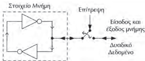
Σχήμα 3.5.3 Βασική μονάδα αποθήκευσης στατικής μνήμης
