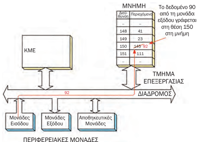
Σχήμα 3.1.12 DMA Μεταφορά
