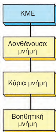
Σχήμα 4.5.1 Επίπεδα μνήμης στον προσωπικό υπολογιστή
