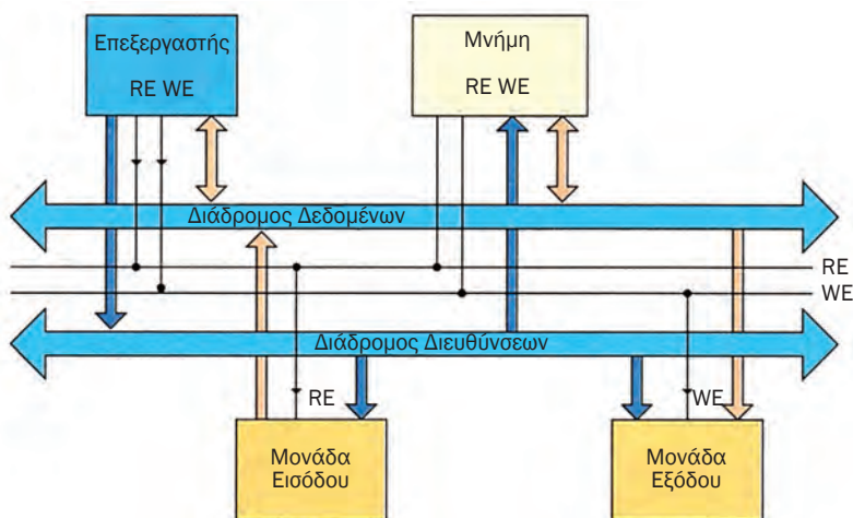
Σχήμα 3.4.3 Διάδρομοι και σήματα ελέγχου
