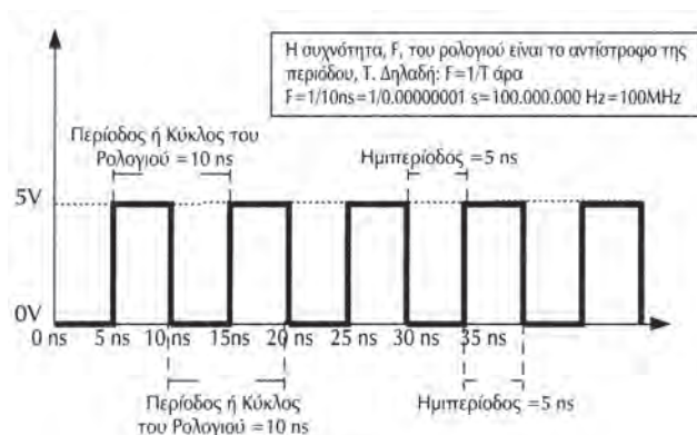
Σχήμα 3.3.1 Η κυματομορφή του ρολογιού συχνότητας 100 MHz
