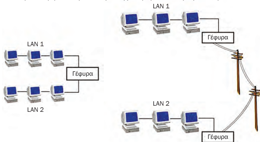
Σχήμα 5.3.9 Γέφυρες
