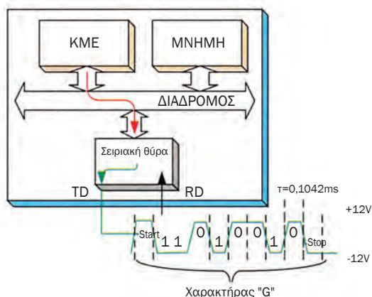
Σχήμα 3.10.2 Η σειριακή θύρα στέλνει δεδομένα
