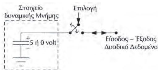
Σχήμα 3.5.3 Βασική μονάδα αποθήκευσης δυναμικής μνήμης
