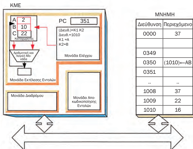
Σχήμα 3.2.9 Η εκτέλεση της εντολής
