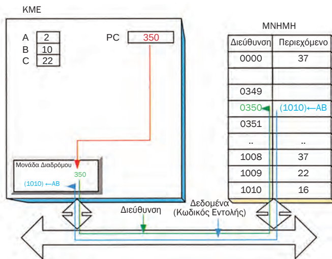
Σχήμα 3.2.4 Μονάδα Διαδρόμου
