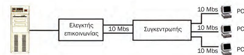
Σχήμα 5.3.8 Η χρήση ενός συγκεντρωτή
