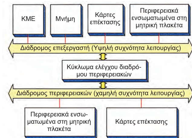
Σχήμα 4.6.4 Διάγραμμα τοπικού διαδρόμου προσωπικού υπολογιστή
