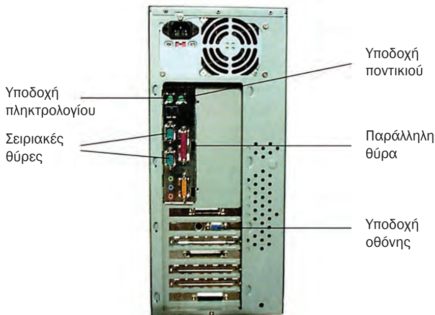
Σχήμα 4.1.6 Πίσω όψη της κεντρικής μονάδας του προσωπικού υπολογιστή
