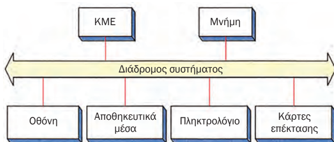
Σχήμα 4.1.2 Βασική αρχιτεκτονική προσωπικού υπολογιστή
