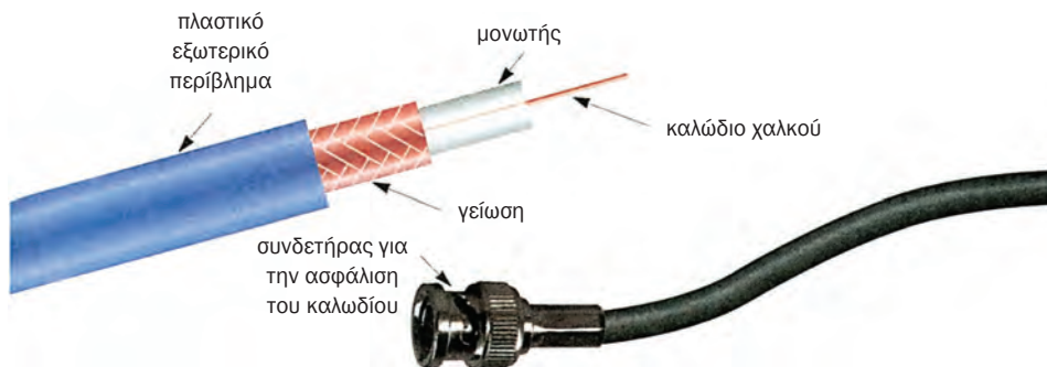
Σχήμα 5.2.8 Ομοαξονικό καλώδιο
